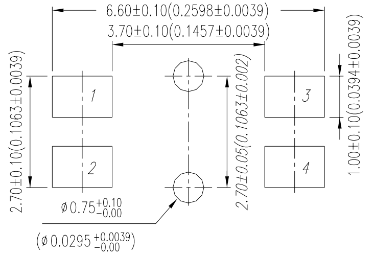
P.C.B LAYOUT
